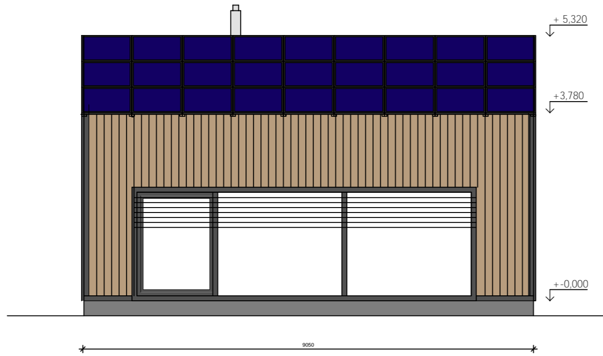
Pohled Jih
