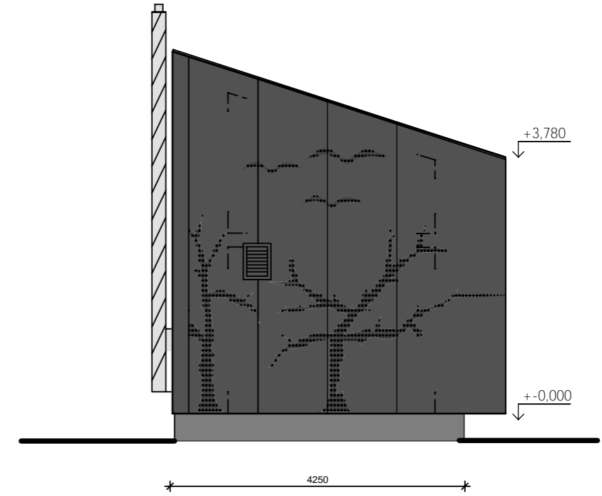
Pohled Západ
