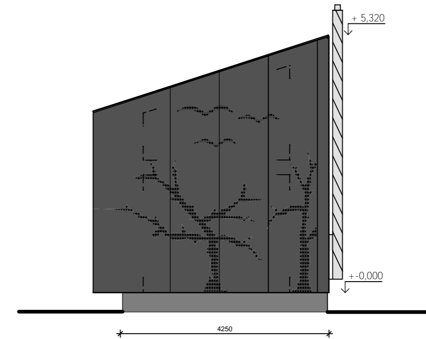
Pohled Východ
